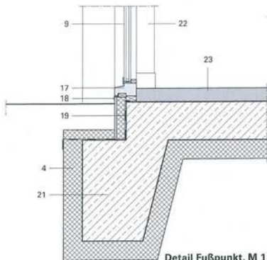
Detail Fußpunkt, M 1:20
